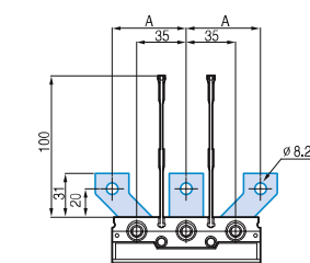
TS100, 160, 250 3P
