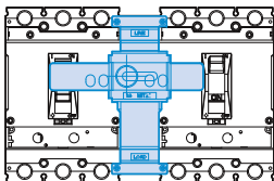
Левый выключатель: ОТКЛ заблокировано Правый выключатель: ВКЛ/ ОТКЛ возможно
