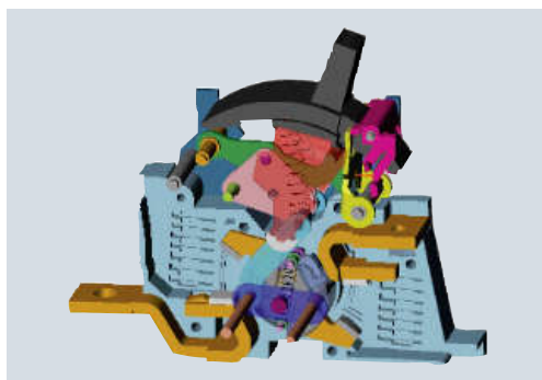
Рис. 4. Положение «ОТКЛ.»
