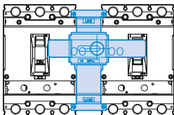
Левый выключатель: ВКЛ/ОТКЛ возможно Правый выключатель: ОТКЛ заблокировано
