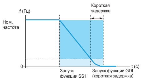
Действие функции безопасности GDL (пример останова: SS1)
